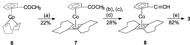
Scheme 1. Preparation of 3 : a) 1,8-cyclododecadiyne; b) LDA/THF; c) ClPO(OEt) 2 ; d) LDA, HCl; e) Cu(OAc) 2 , pyridine
