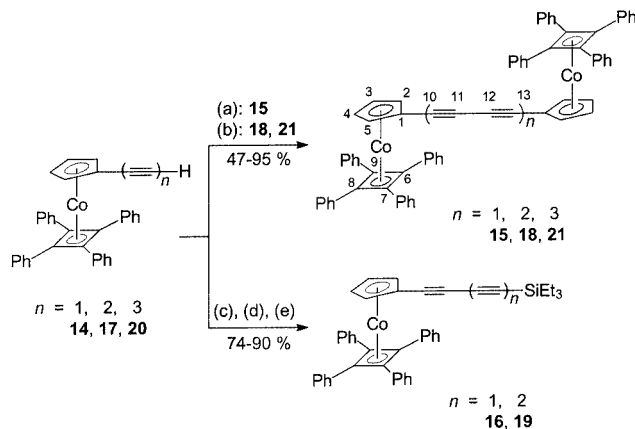
Scheme 3. Synthesis of 15 , 16 , 18 , 19 , 21 : a) CuCl/pyridine + O 2 ; b) CuCl/TMEDA + O 2 ; c) n BuLi; d) CuCl; e) Br-C≡C-SiMe 3 , EtNH 2
