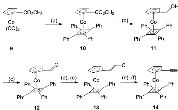
Scheme 2. Preparation of 14 : a) toluene, xylene, 120 °C; b) LiAlH 4 /ether; c) BaMnO 4 ; d) ClCH 2 P(C 6 H 5 ) 3 + Cl - ; e) KOtBu; f) C 6 H 5 Li
